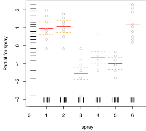
Figure 14: Reprezentarea grafica a rezultatelor functiei aov cu termplot() .
