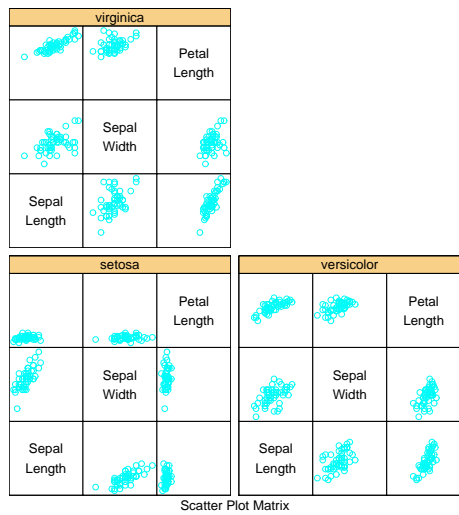
Figure 11: Functia splom cu setul de date “iris” (2).
